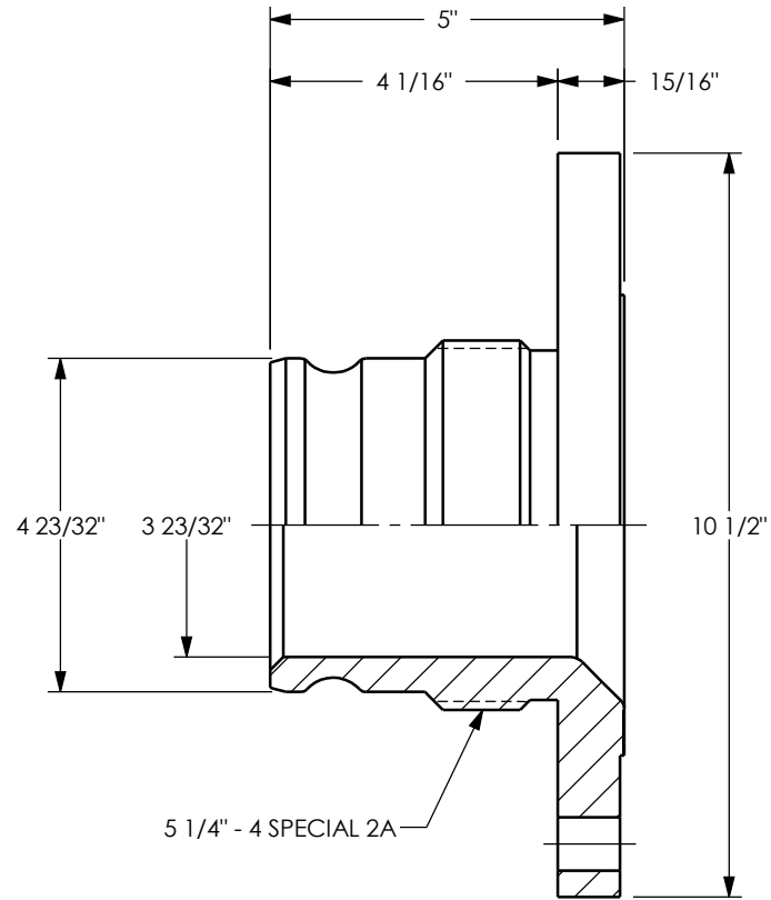
SECTION A-A
